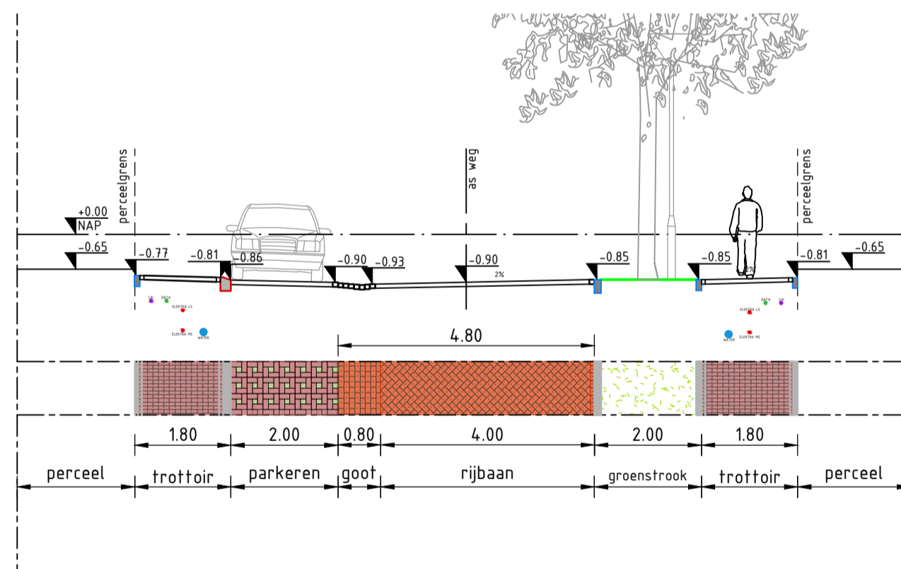
DOORSNEDE C-C Schaal 1:100 Nigtevechtlaan
