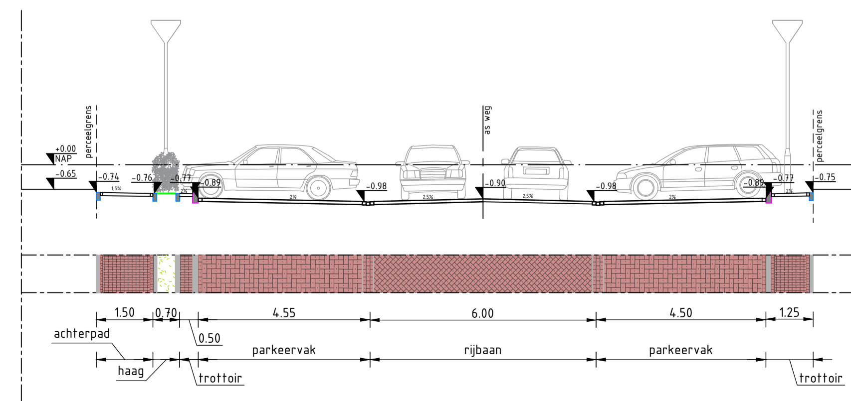
DOORSNEDE L-L Schaal 1:100 Parkeerkoffer
