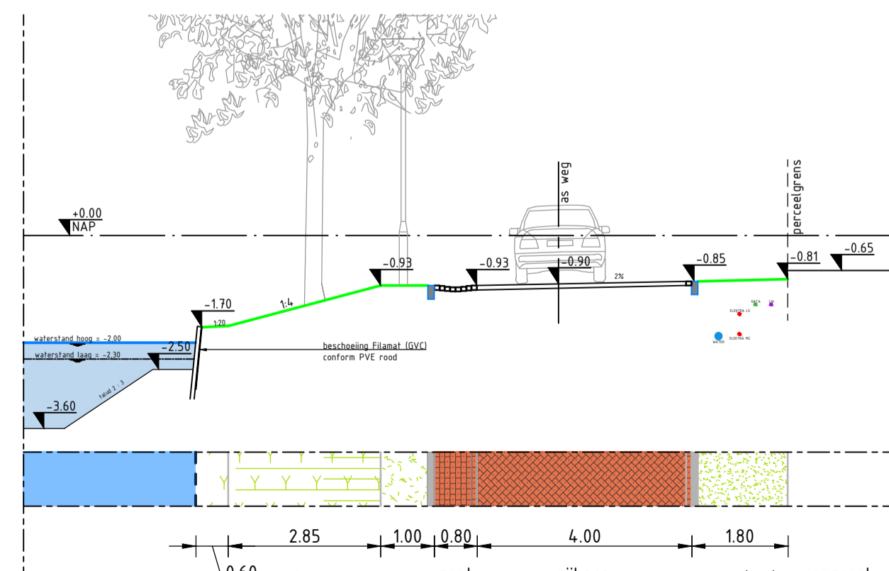
DOORSNEDE H-H Schaal 1:100 Nigtevechtpad
