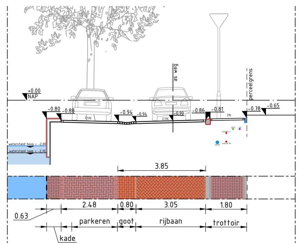
DOORSNEDE D-D Schaal 1:100 Nigtevechtkade
