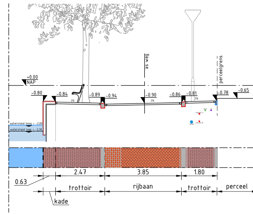
DOORSNEDE E-E Schaal 1:100 Nigtevechtkade
