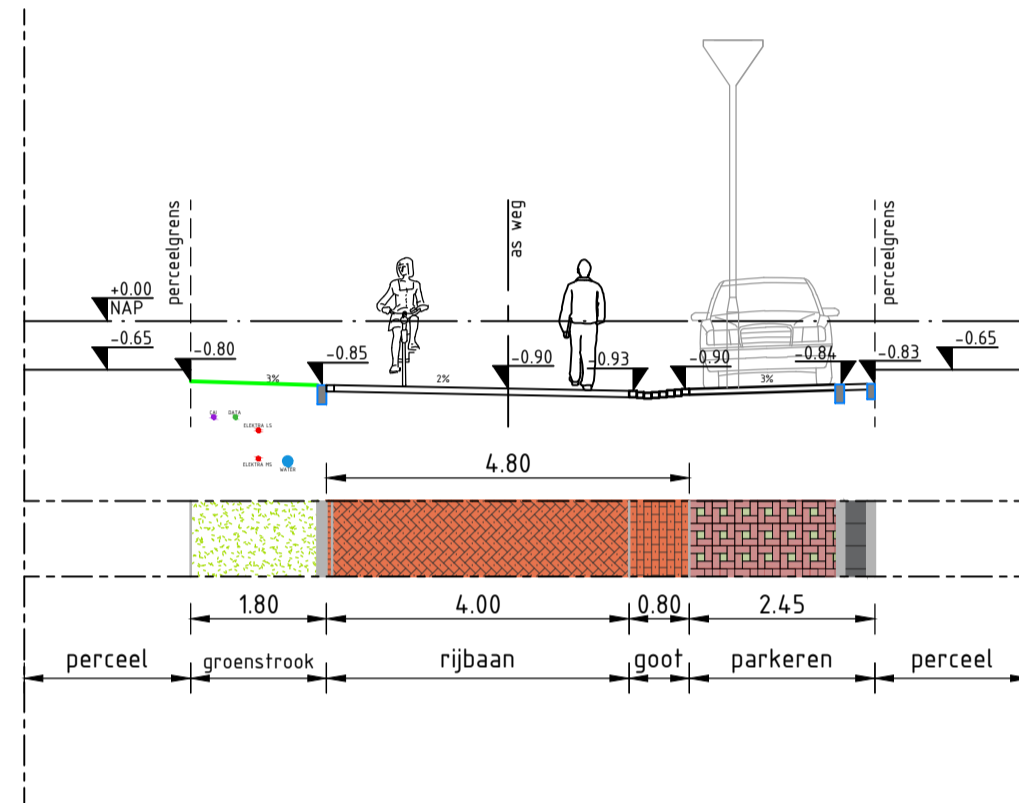
DOORSNEDE B-B Schaal 1:100 Nigtevechtlaan/Nigtevechtstraat
