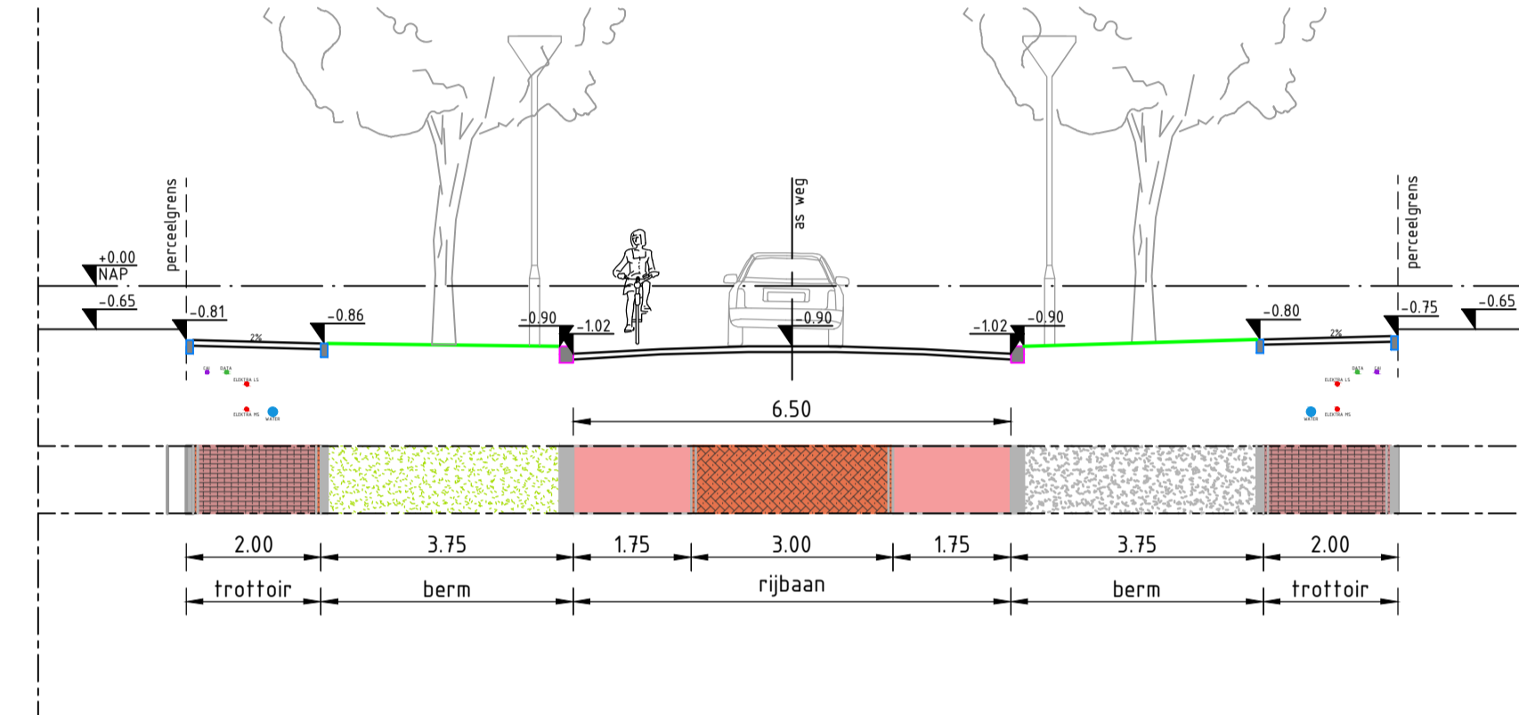
DOORSNEDE J-J Schaal 1:100 Vechtsroomlaan
