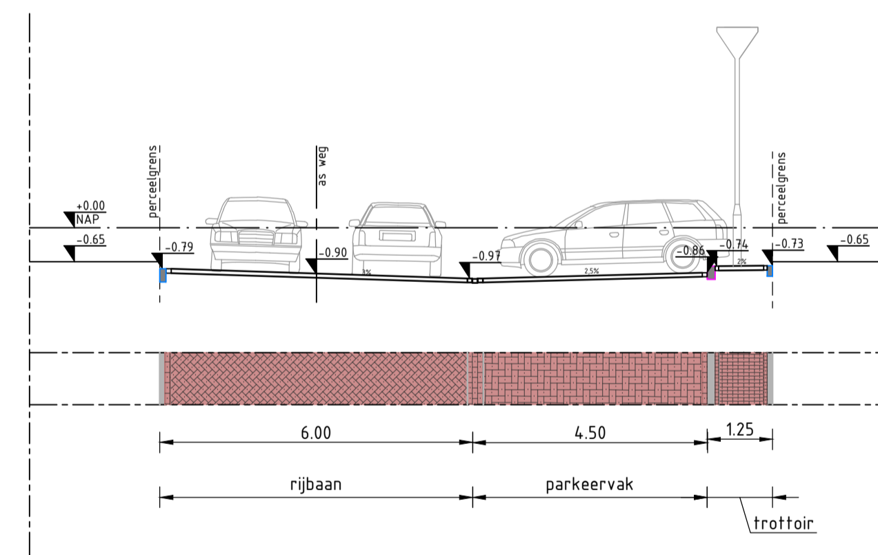
DOORSNEDE K-K Schaal 1:100 Parkeerkoffer
