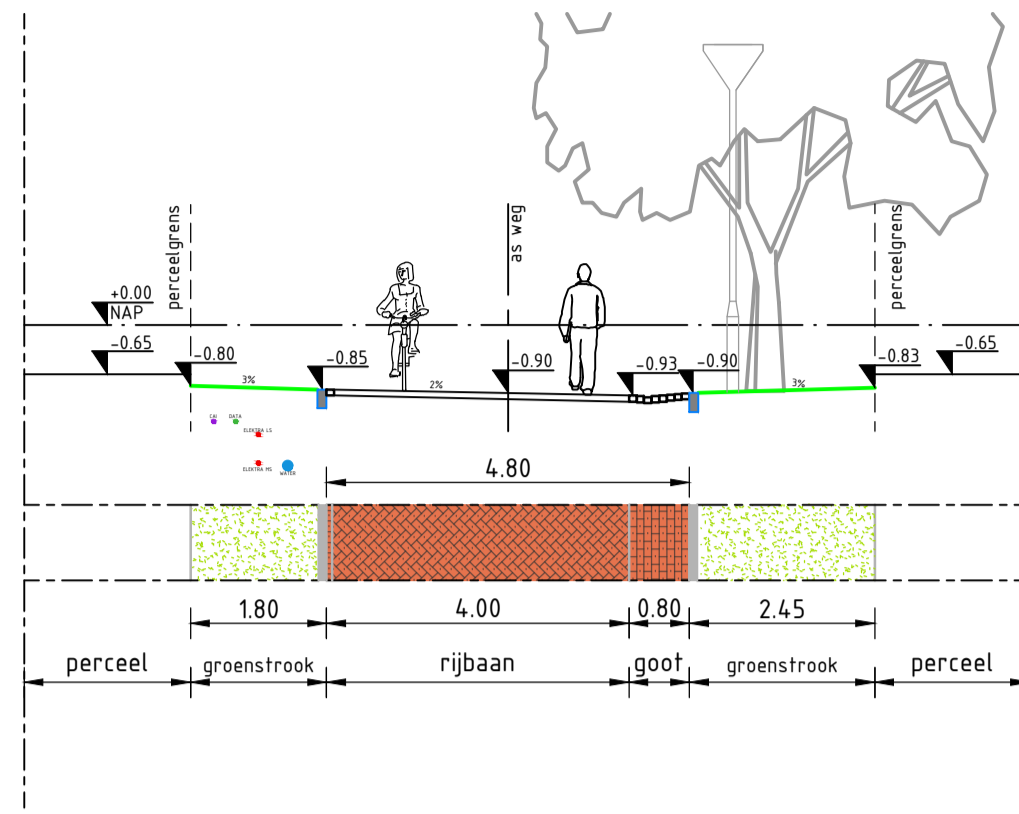
DOORSNEDE A-A Schaal 1:100 Nigtevechtlaan/Nigtevechtstraat
