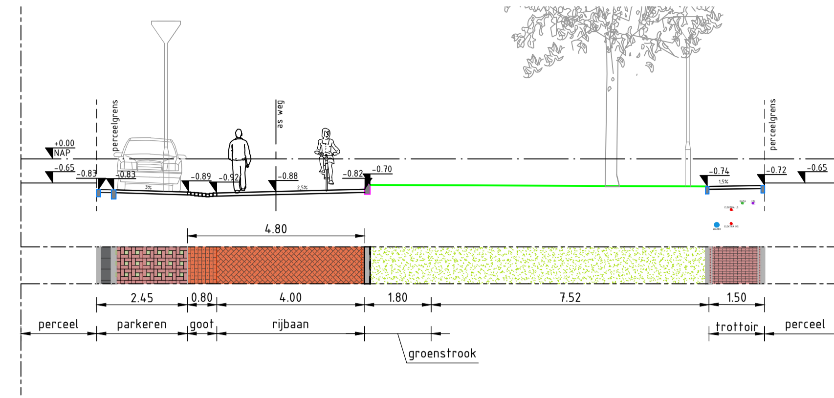
DOORSNEDE I-I Schaal 1:100 Nigtevechtpad
