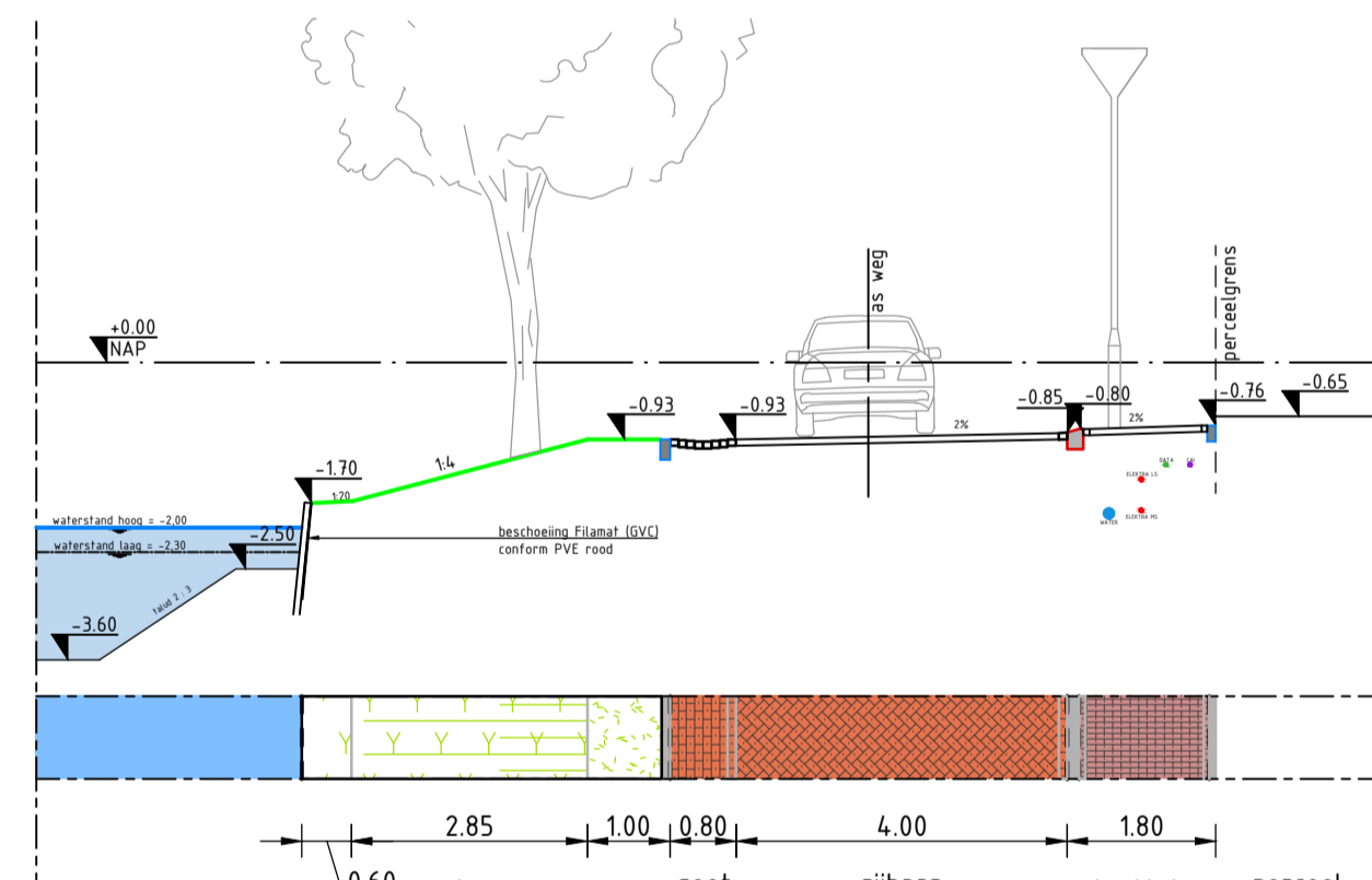
DOORSNEDE G-G Schaal 1:100 Nigtevechtlaan
