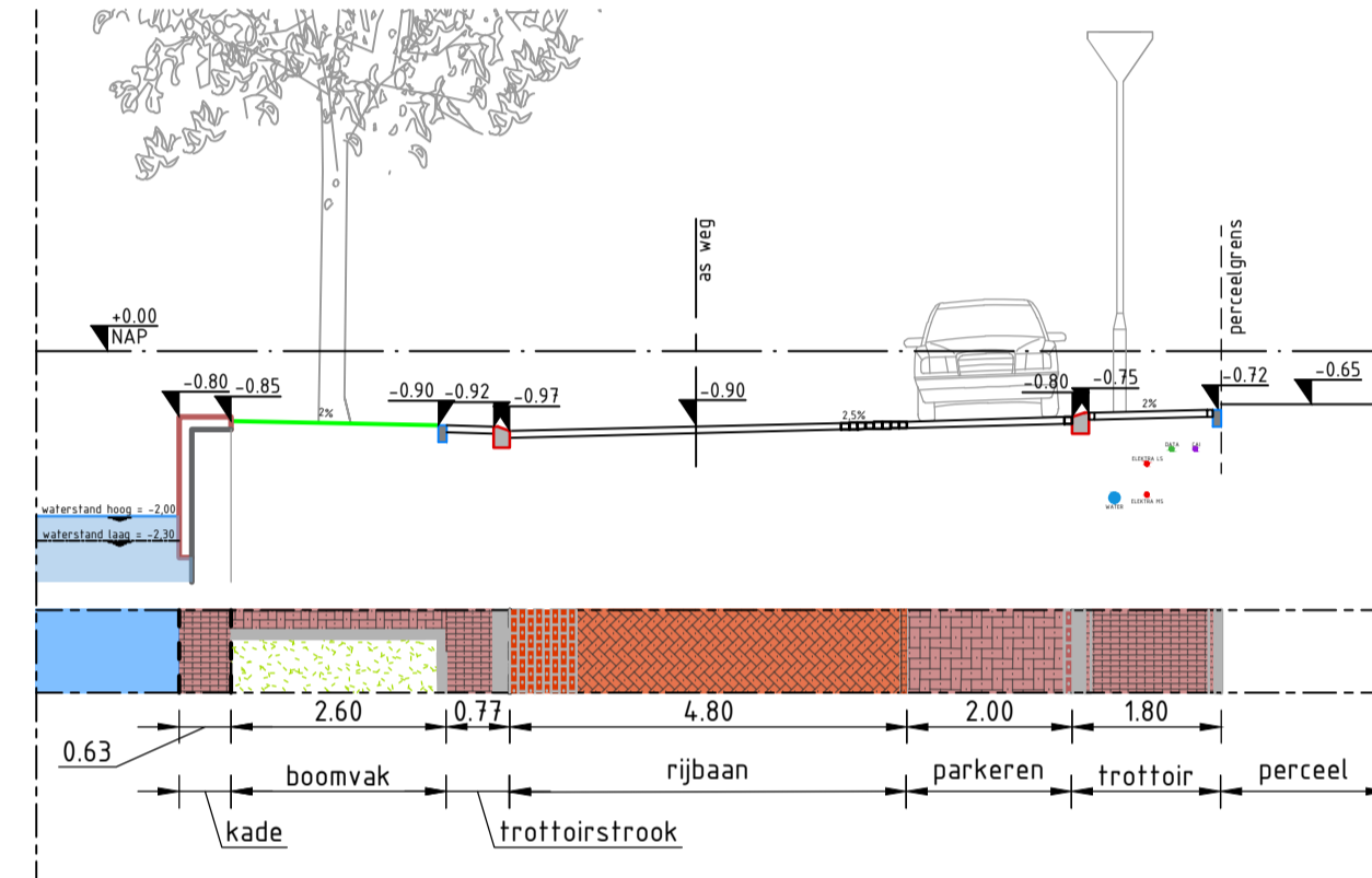
DOORSNEDE F-F Schaal 1:100 Nigtevechtlaan
