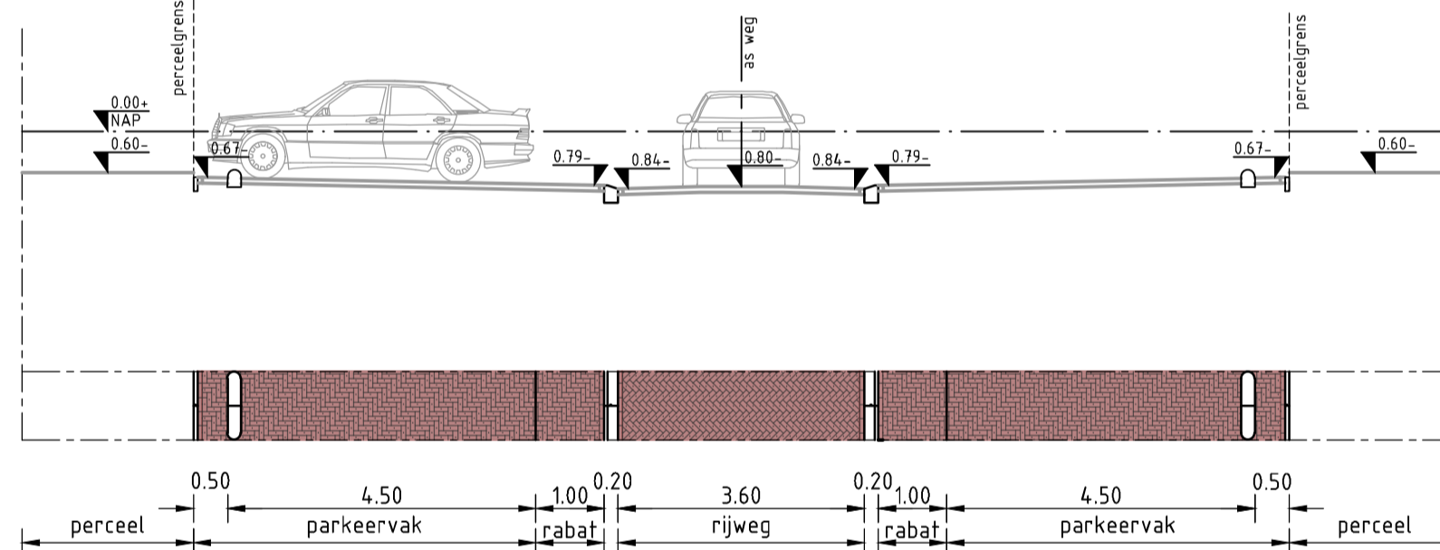
Doorsnede H-H schaal 1:100
