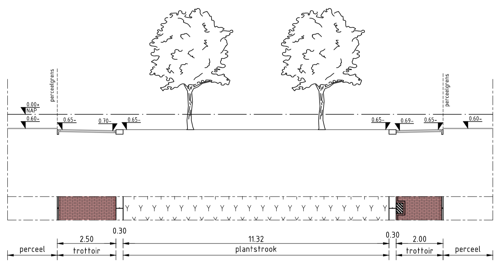
Doorsnede G-G schaal 1:100
