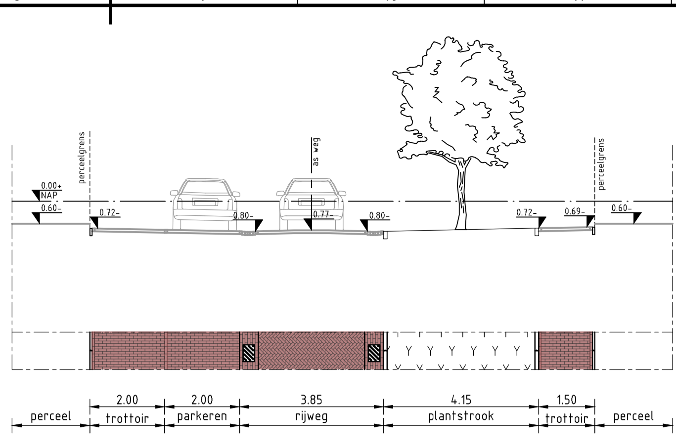
Doorsnede F-F schaal 1:100
