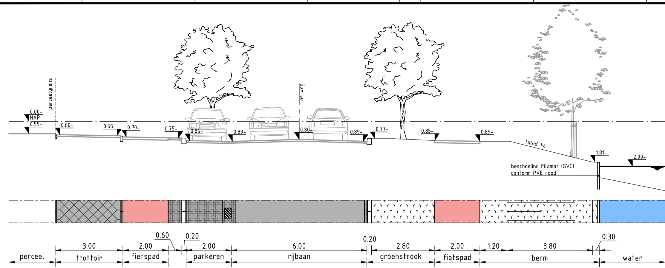
Doorsnede A-A schaal 1:100
