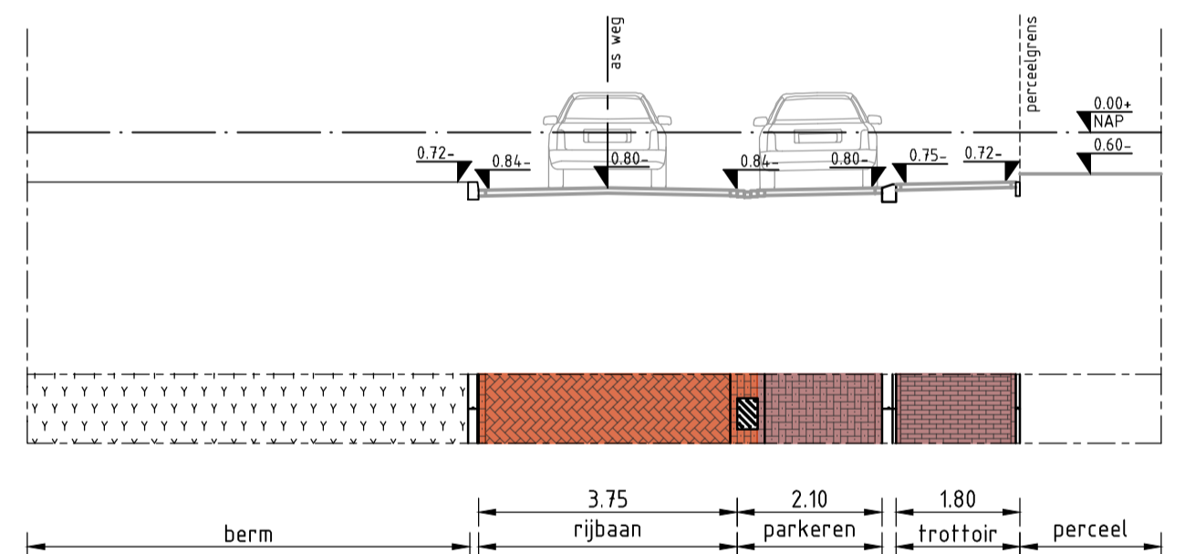
Doorsnede C-C schaal 1:100
