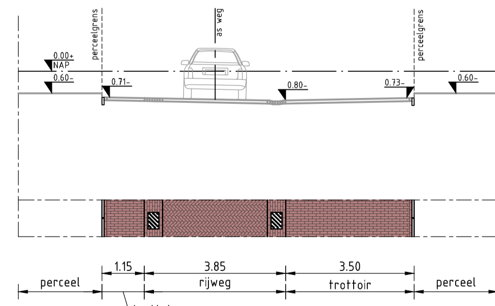
Doorsnede E-E schaal 1:100
