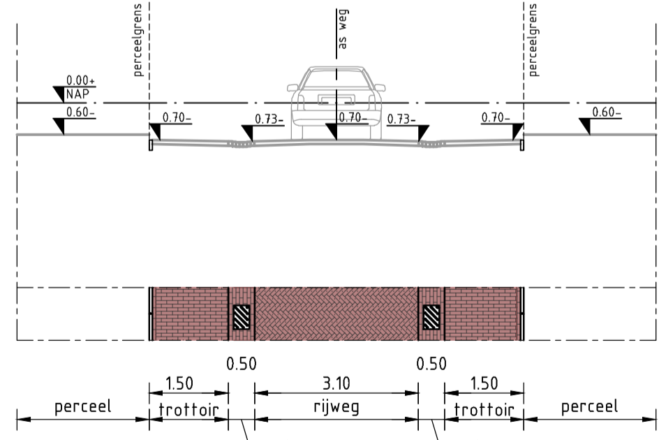
Doorsnede I-I schaal 1:100
