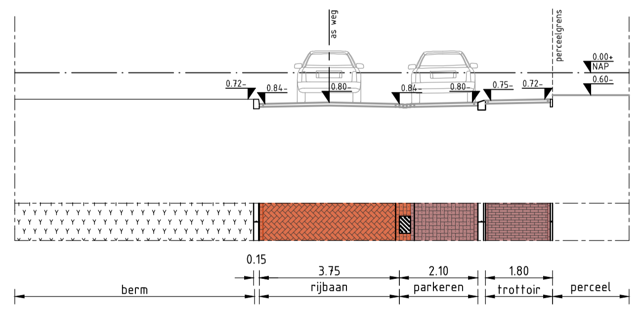
Doorsnede D-D schaal 1:100
