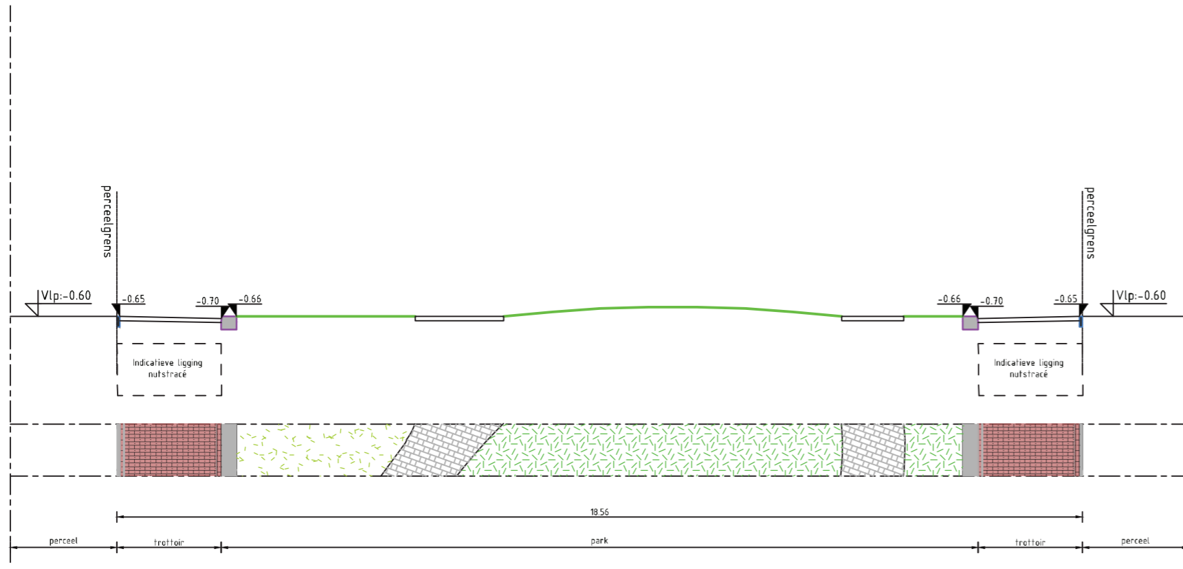
Profiel G-G
