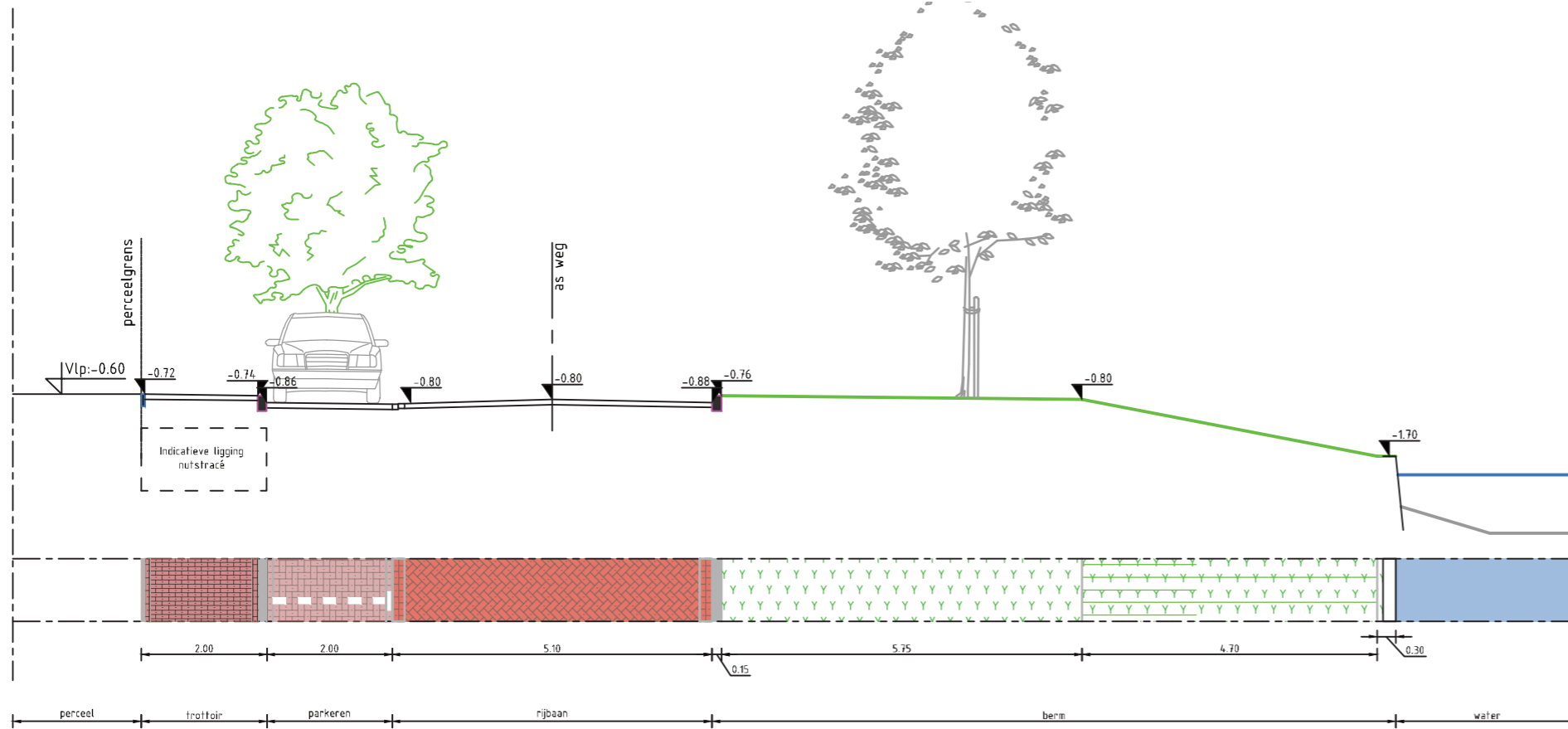
Profiel A-A
