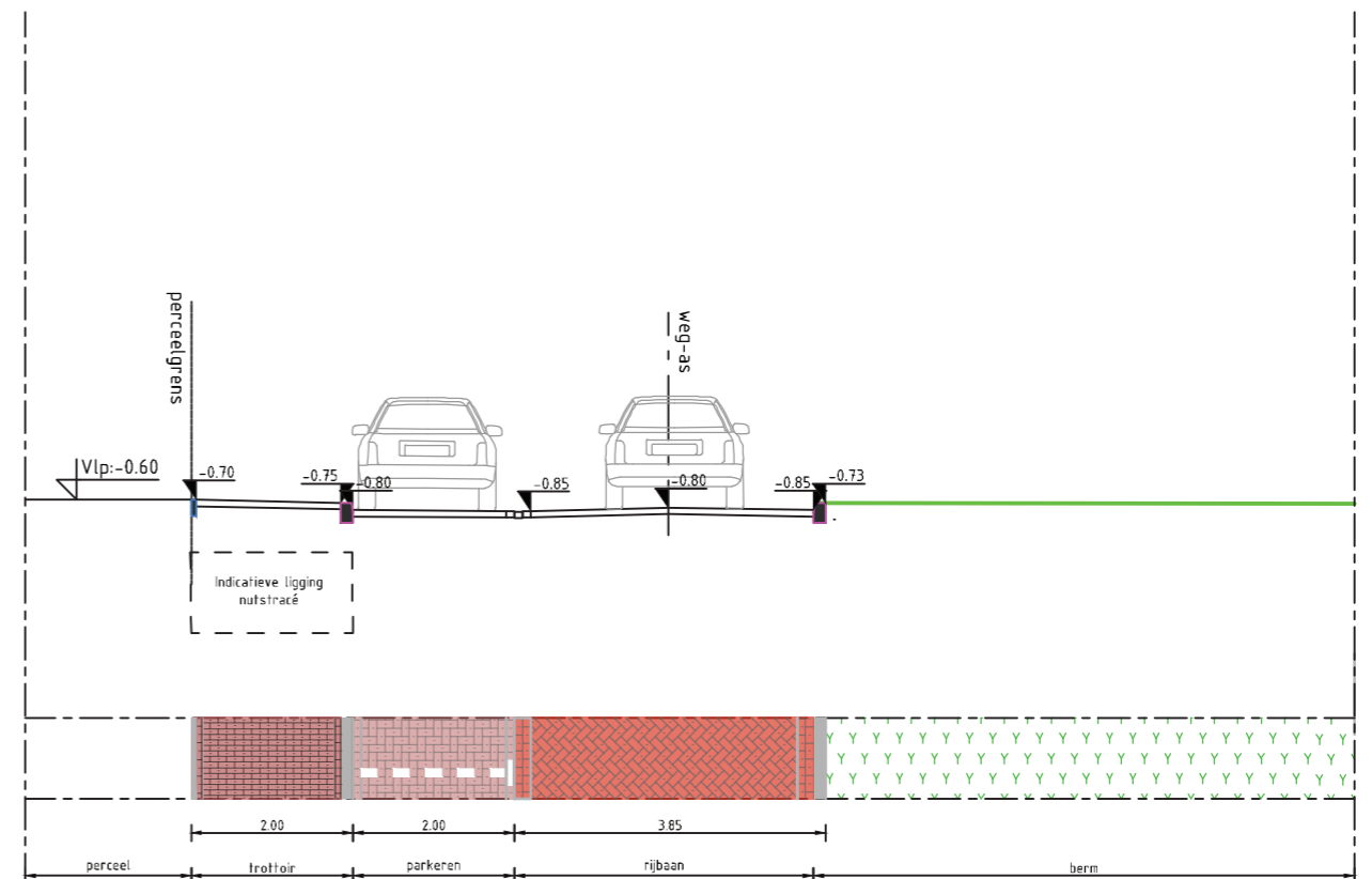
Profiel C-C
