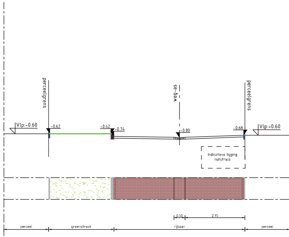
Profiel F-F
