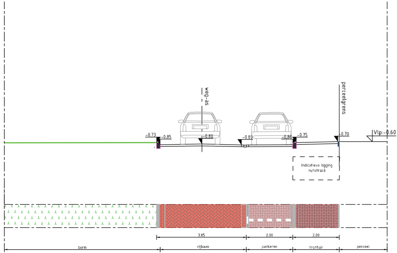
Profiel D-D
