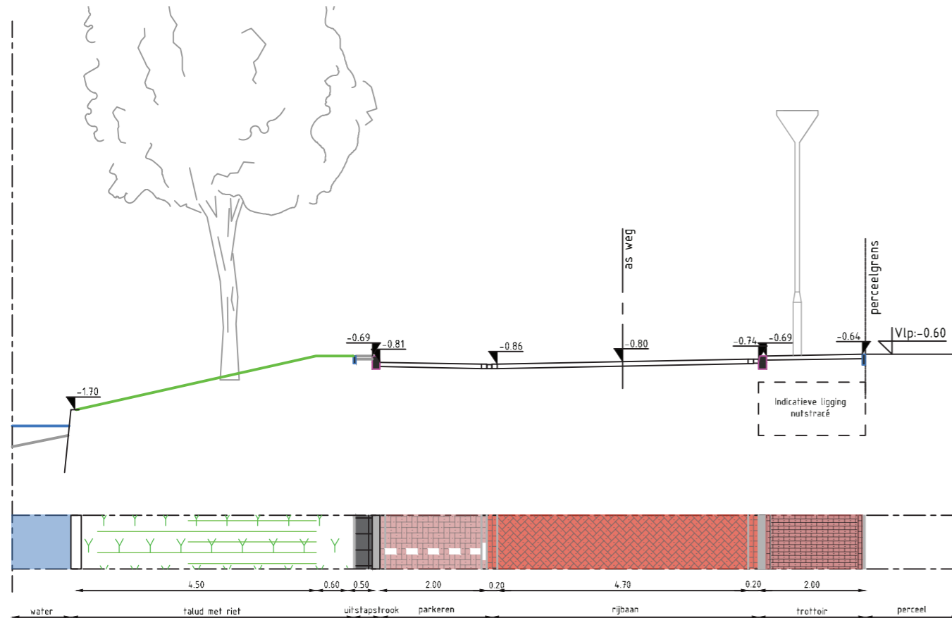
Profiel B-B
